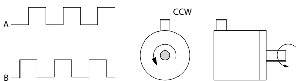
Disegno 12.6 Individuazione della direzione dell'encoder
