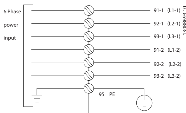
Disegno 10.3 Collegamento della rete, frame F8-F13
