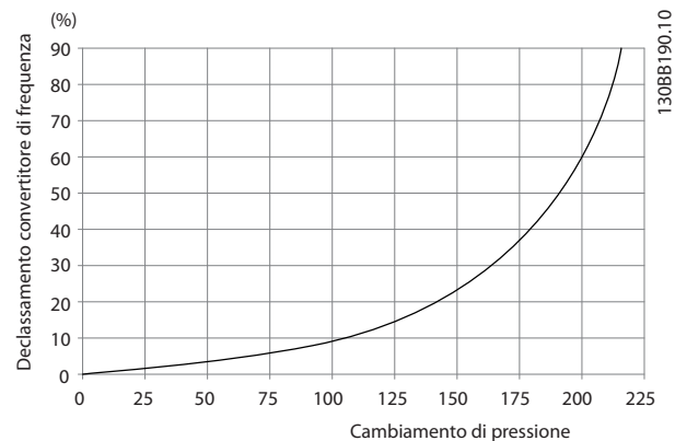
Disegno 9.7 Declassamento rispetto alla variazione di pressione per frame F1-F4. Flusso d'aria: 580 cfm (985 m 3 /h)
