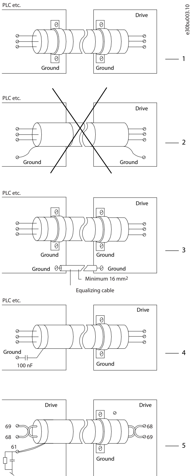
Disegno 10.7 Esempi di messa a terra
